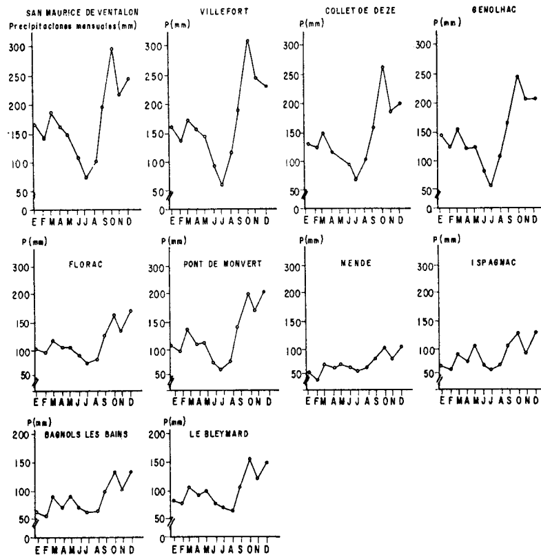
Fig. 3. Curvas de precipitaciones mensuales de las 10 estaciones.
