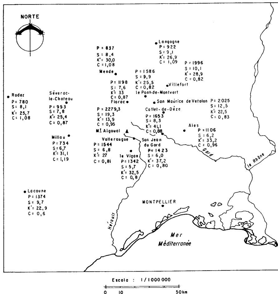
Fig. 9. Los valores de precipitación anual (P), índice de sequía estival (S), continentalidad térmica (K), continentalidad pluviométrica (c), para algunas estaciones de la región y sus alrededores.
