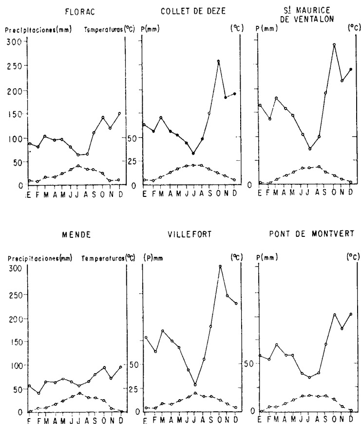
Fig. 8. Los diagramas ombrotérmicos de 6 estaciones.
